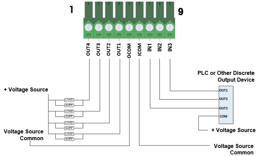
图 A-79: 共地输入和共地输出
