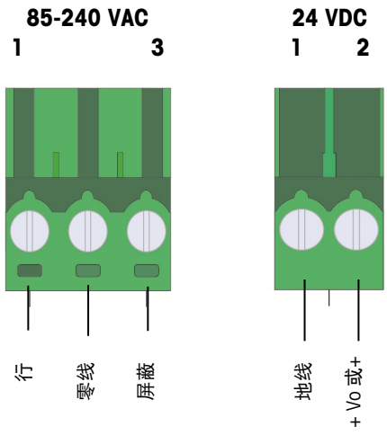
图 A-31: 输入电源连接
