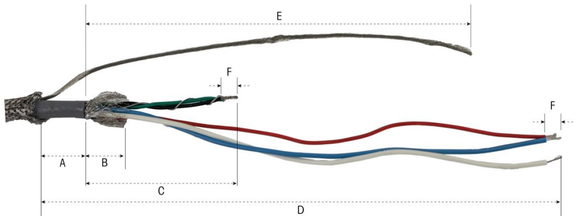
图 A-50：POWERCELL 电缆准备-防尘式
