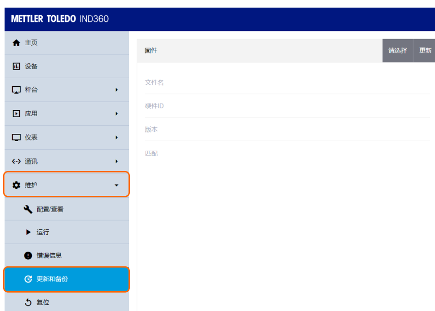
图 4-5: 更新和备份菜单
