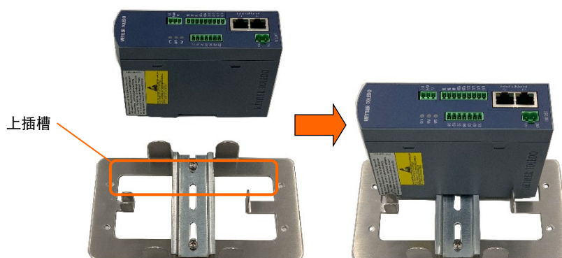
图 A-14: 称重仪表模块安装
