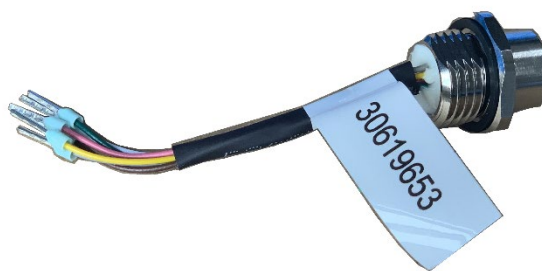
图 A-47: M12 到接线端子转接线(30619653)
