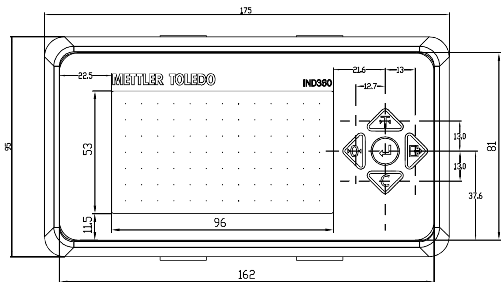
图 1-11: IND360 面板式正面尺寸图
