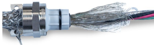
图 A-53: 内部屏蔽层已解开
