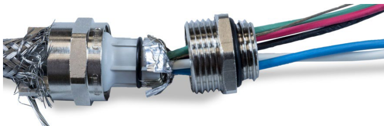
图 A-57：接头主体准备就绪，可安装在索环上方
