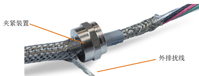
图 A-51: 接头外部已安装在电缆上
