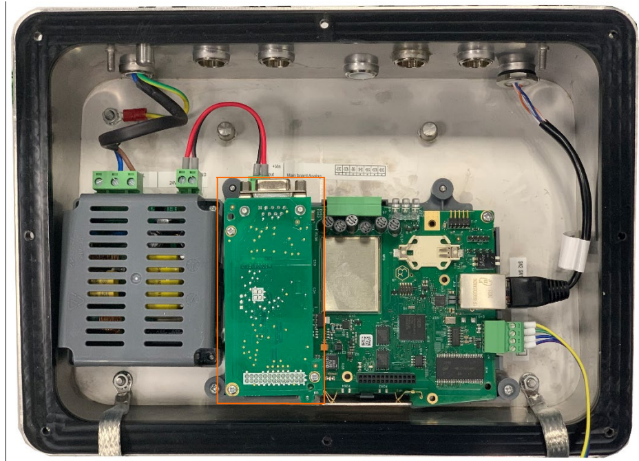
图 A-88: PROFIBUS DP 选件板, 已安装
