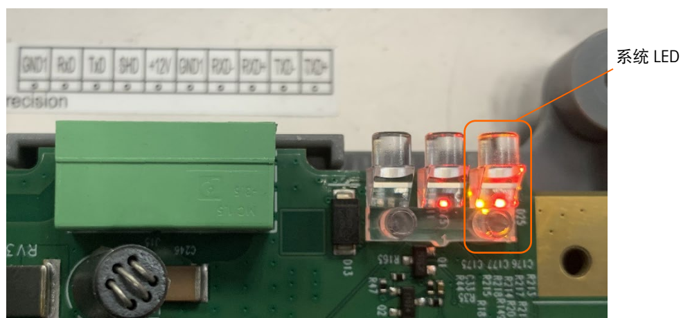
图 4-20: 系统 LED 位置
