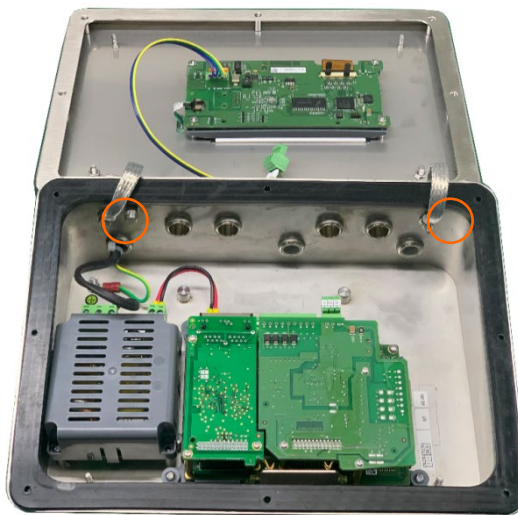
图 A-22：前面板已反转
