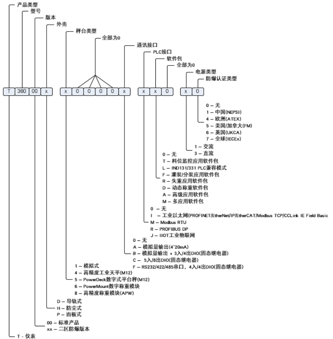
图 1-7: IND360 SCK 标识
