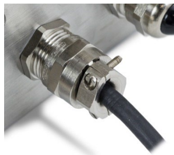
图 A-70: 接头已安装
