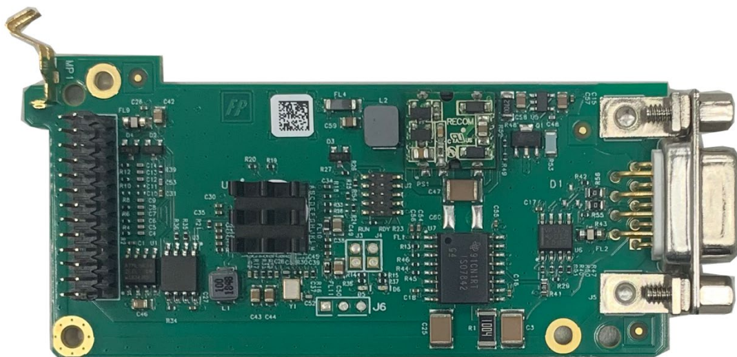
图 A-87: PROFIBUS DP 选件板
