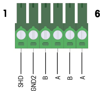
图 A-89: Modbus RTU 选件板
