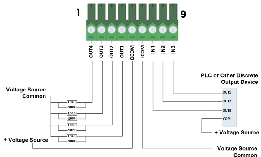
图 A-78: 共地输入和共源输出
