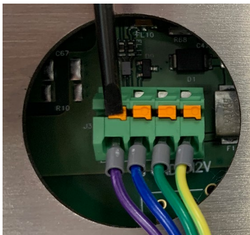
图 A-17: 显示电缆连接器上的橙色压块
