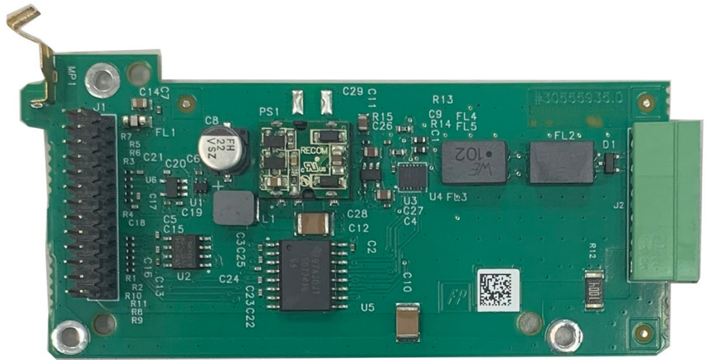
图 A-89: Modbus RTU 选件板
